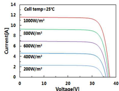
放射照度特性 (I-V) : LR6-600PH-345M
