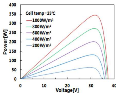
放射照度特性 (P-V) : LR6-600PH-345M
