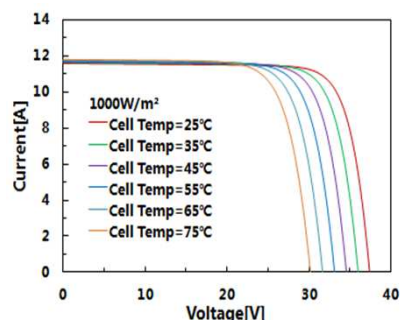
温度特性 (I-V) : LR6-600PH-345M
