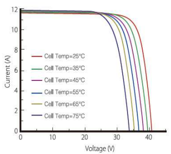
温度特性 (I-V) : LR4-60HPH-365M
