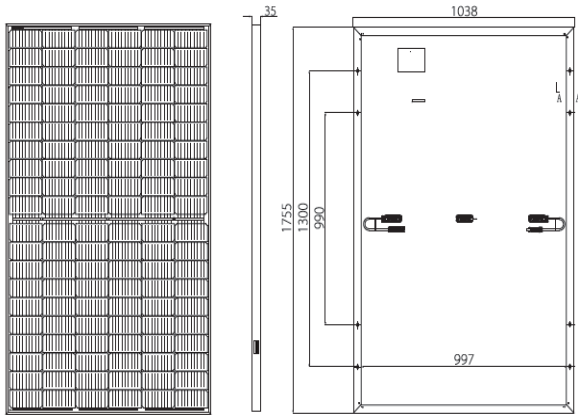
単位：mm 公差：長辺 ±2mm, 短辺 ±2mm 厚さ ±1mm, 穴ピッチ ±1mm
